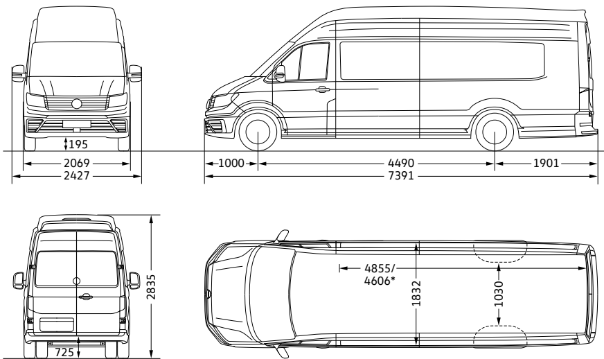
Crafter 50 Skriňová dodávka dlhý rázvor s previsom so super vysokou strechou
