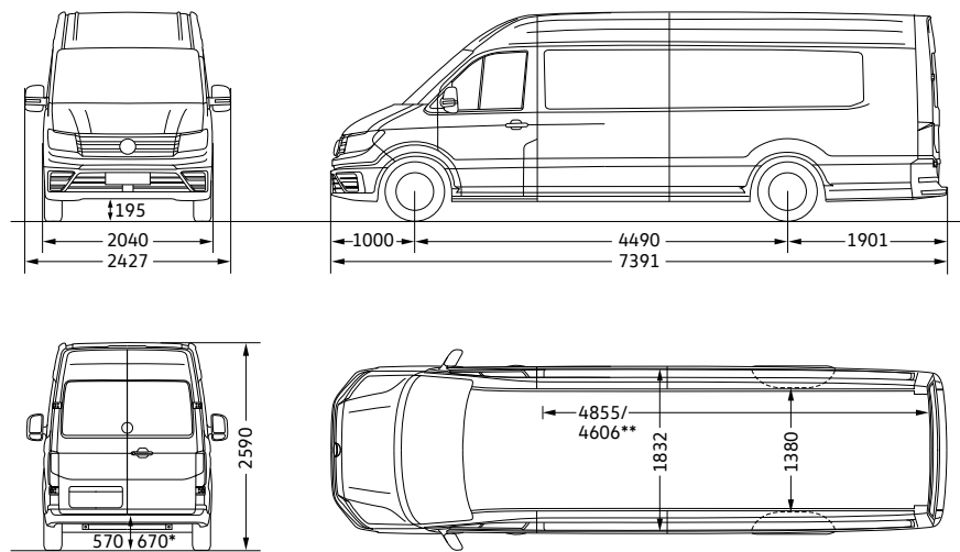
Crafter 35 Skriňová dodávka dlhý rázvor s previsom s vysokou strechou
