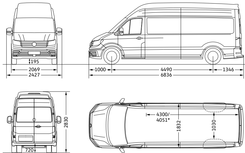
Crafter 50/55 Skriňová dodávka dlhý rázvor so super vysokou strechou
