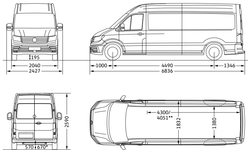
Crafter 35 Skriňová dodávka dlhý rázvor s vysokou strechou
