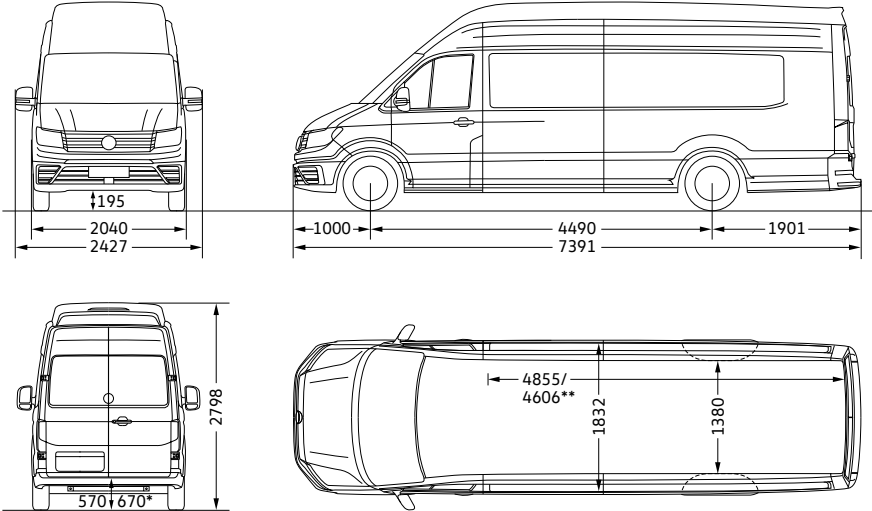
Crafter 35 Skriňová dodávka dlhý rázvor s previsom so super vysokou strechou
