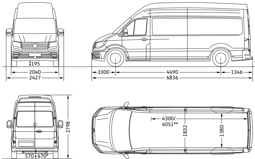
Crafter 35 Skriňová dodávka dlhý rázvor so super vysokou strechou
