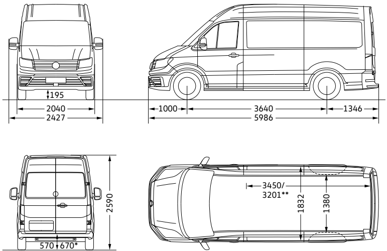
Crafter 35 Skriňová dodávka krátky rázvor s vysokou strechou
